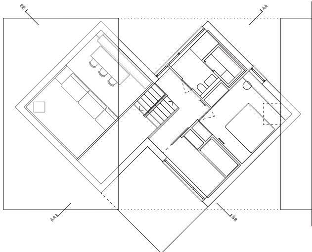
Obergeschoss/ First Floor
