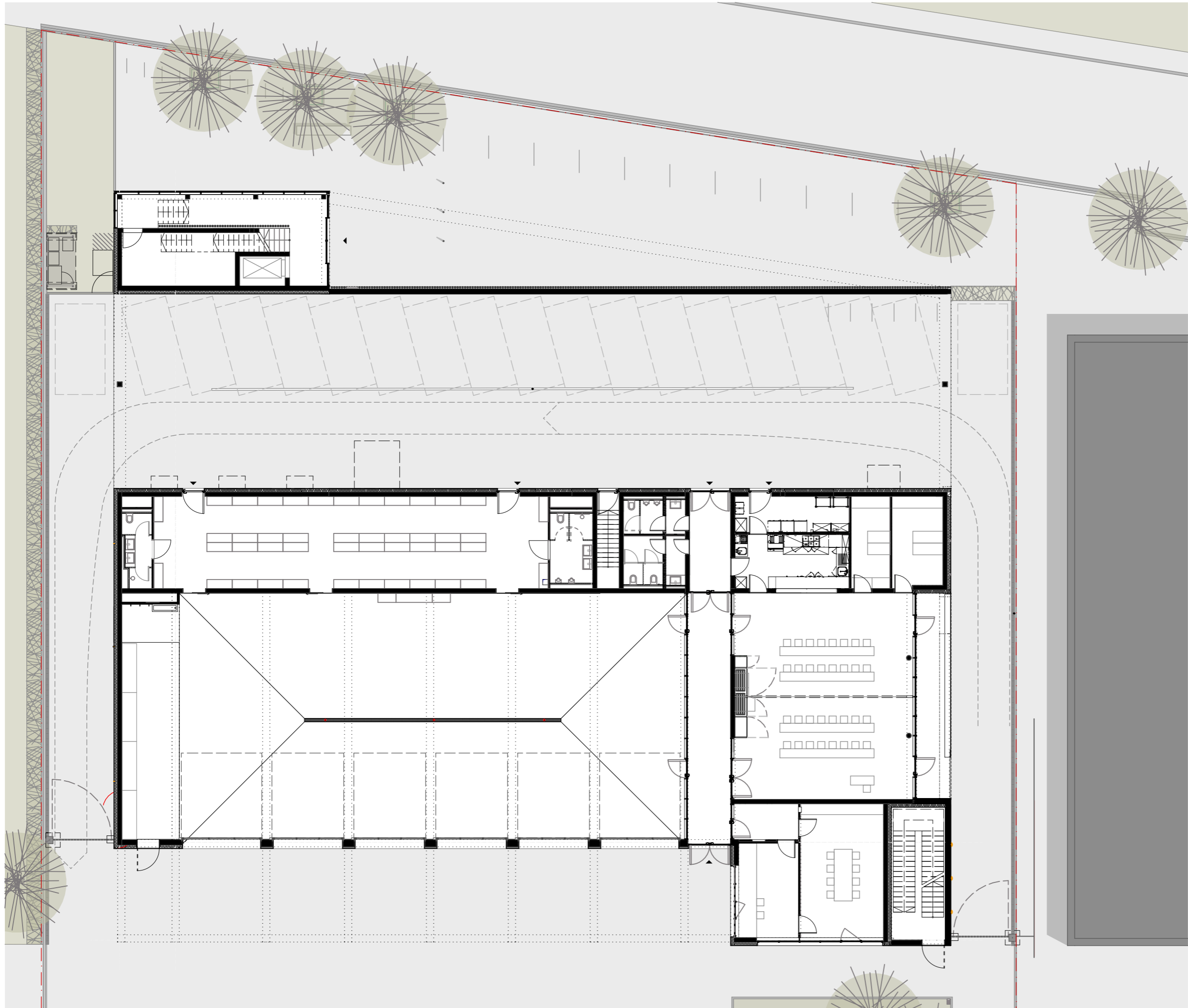
erdgeschoss
